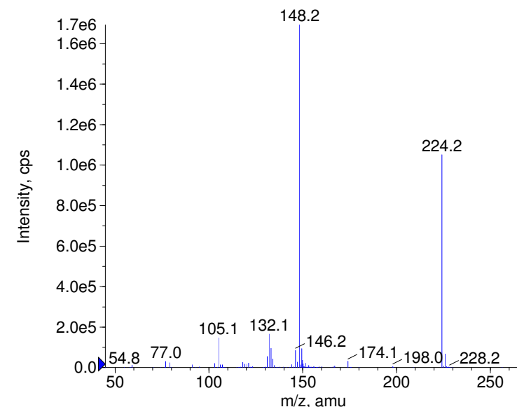
+ Dimethachlor Prec(256.0) CE(99.0) RT(1.1)
