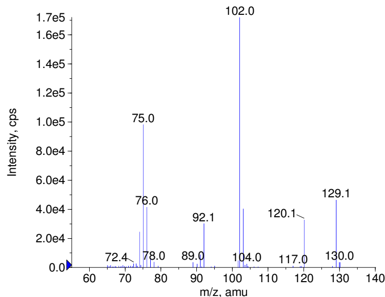
+ Dihydralazine Prec(191.0) CE(50.0) RT(0.8)
