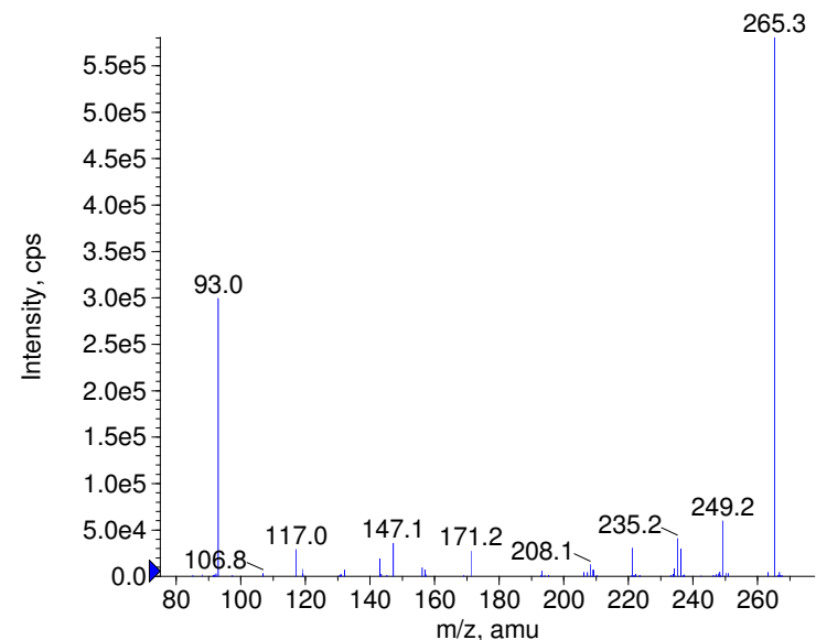
■ - Dienestrol Prec(265.0) CE(-99.0) RT(0.9)
