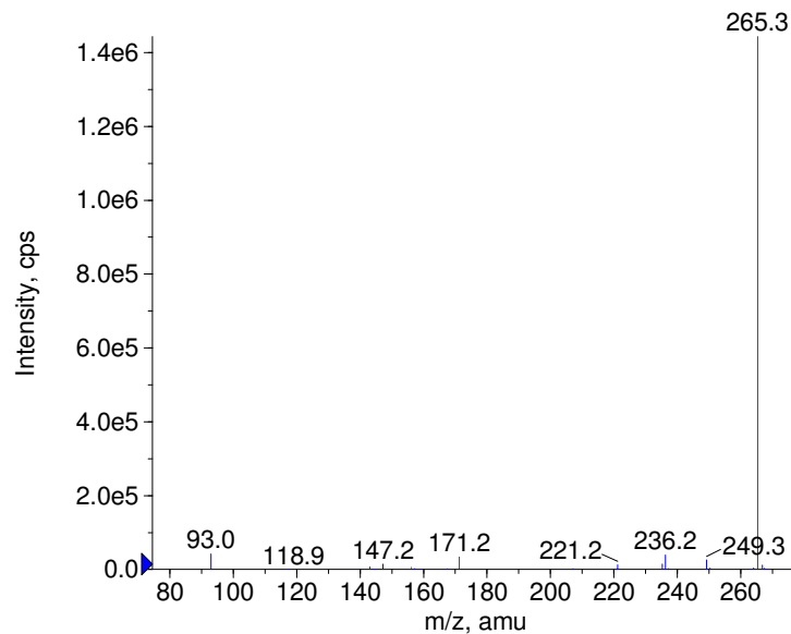
■ - Dienestrol Prec(265.0) CE(-50.0) RT(0.9)
