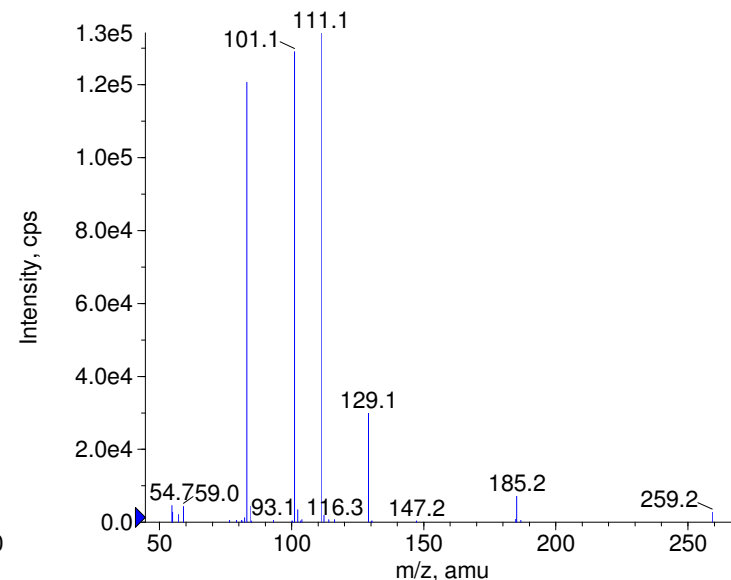
+ Dibutyl adipate Prec(259.0) CE(99.0) RT(3.7)
