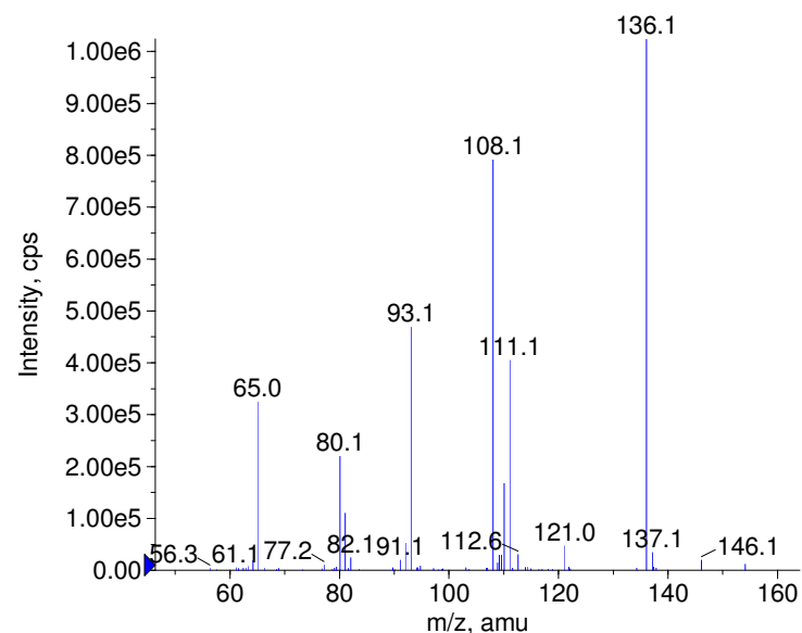
■ + Desmedipham Prec(301.0) CE(50.0) RT(1.3)
