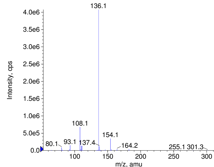
■ + Desmedipham Prec(301.0) CE(99.0) RT(1.3)
