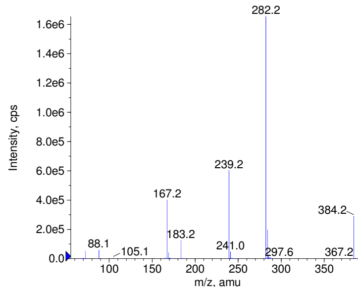
+ Denaverine Prec(384.0) CE(50.0) RT(1.2)
