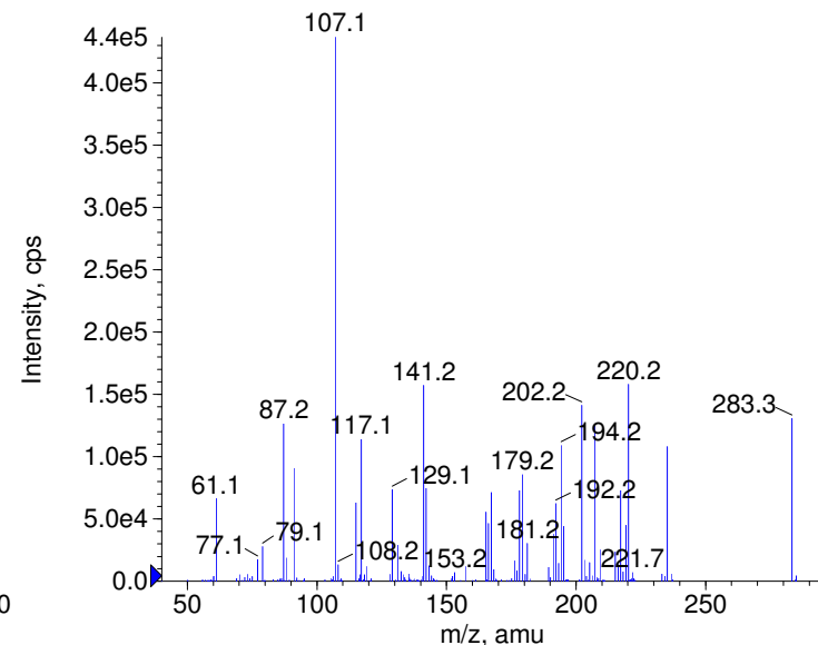
+ D3-Doxepine Prec(283.0) CE(99.0) RT(0.8)
