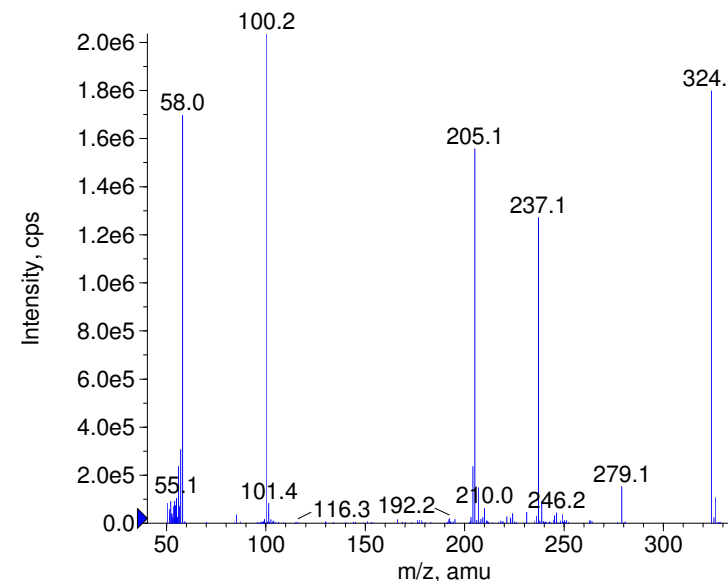
+ Cyamemazine Prec(324.0) CE(99.0) RT(0.9)
