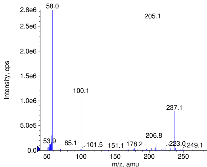
+ Cyamemazine Prec(324.0) CE(50.0) RT(0.9)
