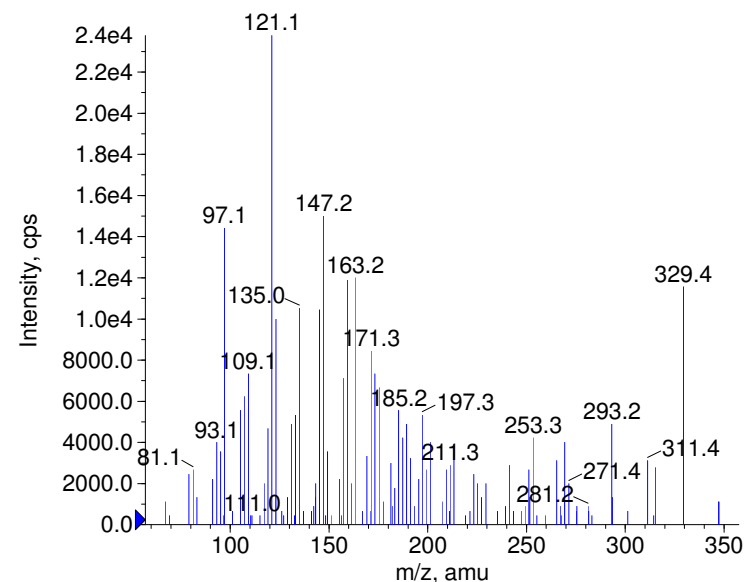
+ Corticosterone Prec(347.0) CE(99.0) RT(1.0)
