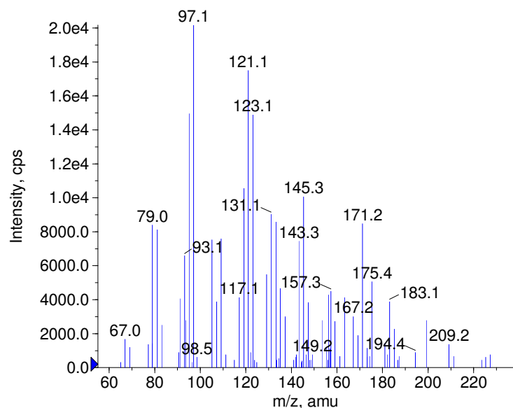
+ Corticosterone Prec(347.0) CE(50.0) RT(1.0)
