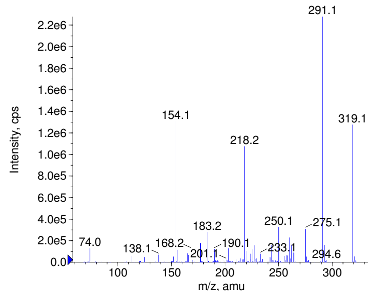
■ + Clotiazepam Prec(319.0) CE(99.0) RT(2.2)
