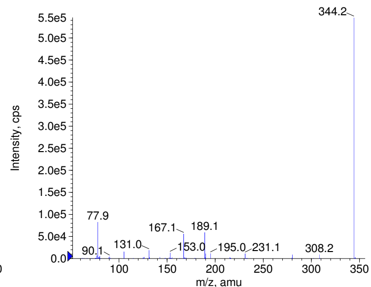
■ - Clopamide Prec(344.0) CE(-99.0) RT(0.9)
