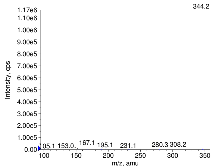
■ - Clopamide Prec(344.0) CE(-50.0) RT(0.8)
