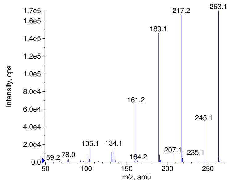
+ Cinoxacin Prec(263.0) CE(99.0) RT(0.9)
