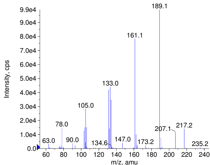
+ Cinoxacin Prec(263.0) CE(50.0) RT(0.9)
