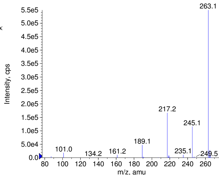
+ Cinoxacin Prec(263.0) CE(50.0) RT(0.9)
