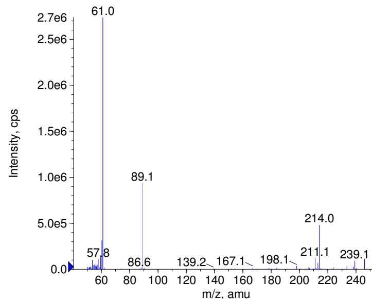
+ Chlorpromazin-D3 Prec(322.0) CE(50.0) RT(0.9)
