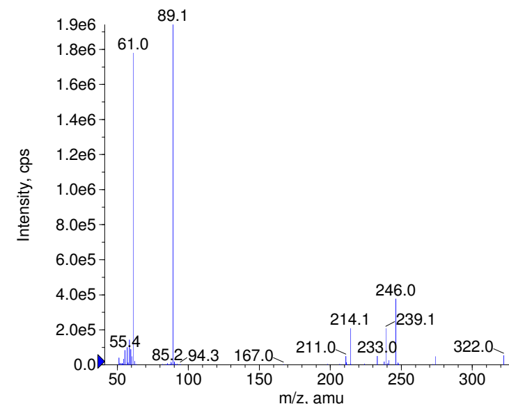
+ Chlorpromazin-D3 Prec(322.0) CE(99.0) RT(0.9)
