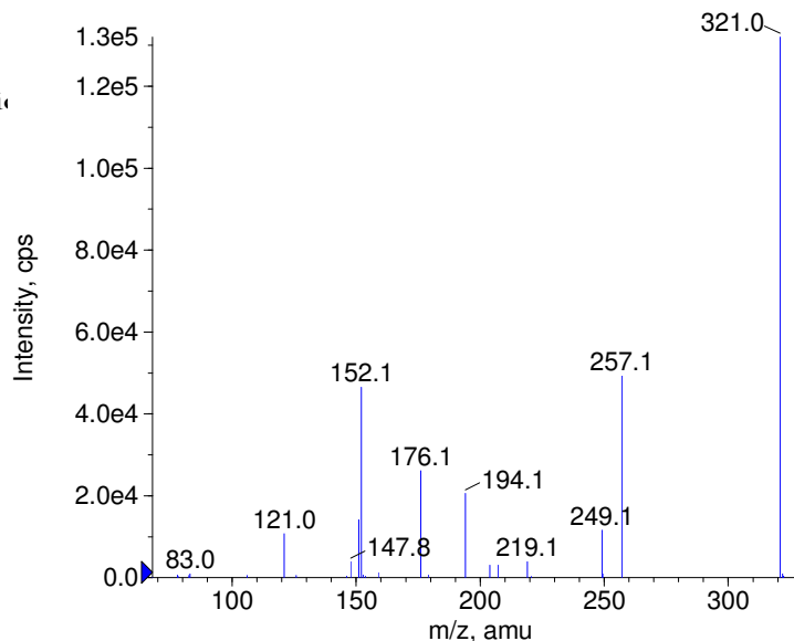
■ - Chloramphenicol Prec(321.0) CE(-50.0) RT(0.9)
