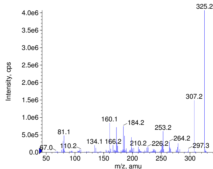
■ + Chinine Prec(325.0) CE(99.0) RT(0.9)
