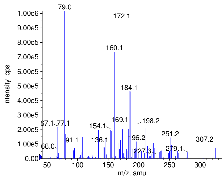
■ + Chinine Prec(325.0) CE(50.0) RT(0.9)
