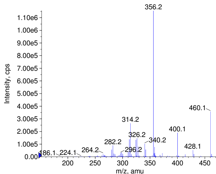
■ + Cerivastatin Prec(460.0) CE(50.0) RT(2.5)
