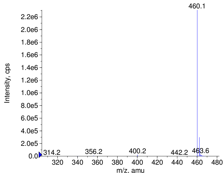
■ + Cerivastatin Prec(460.0) CE(50.0) RT(2.5)
