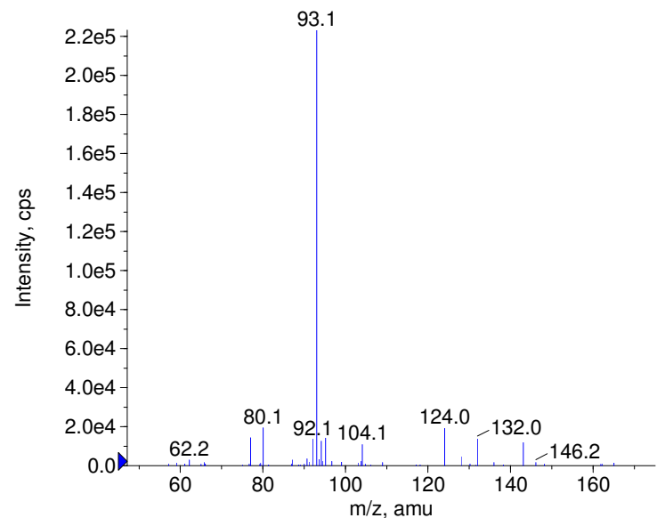
+ Carboxin Prec(236.0) CE(50.0) RT(1.3)
