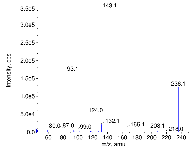
+ Carboxin Prec(236.0) CE(99.0) RT(1.3)
