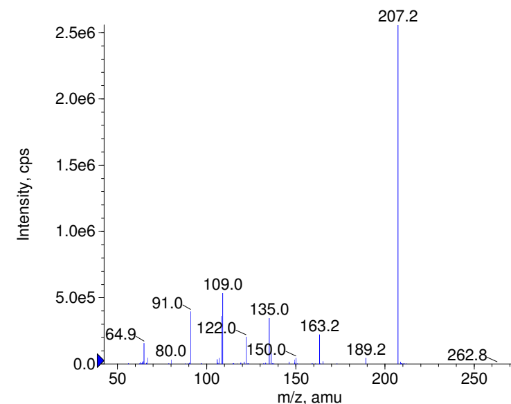
■ - Caproylresorcinol Prec(207.0) CE(-99.0) RT(1.3)
