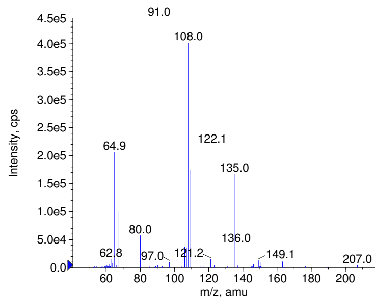
■ - Caproylresorcinol Prec(207.0) CE(-50.0) RT(1.2)
