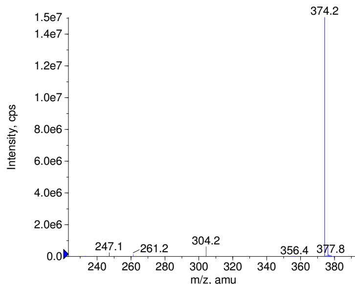
+ Bunazosin Prec(374.0) CE(50.0) RT(0.9)
