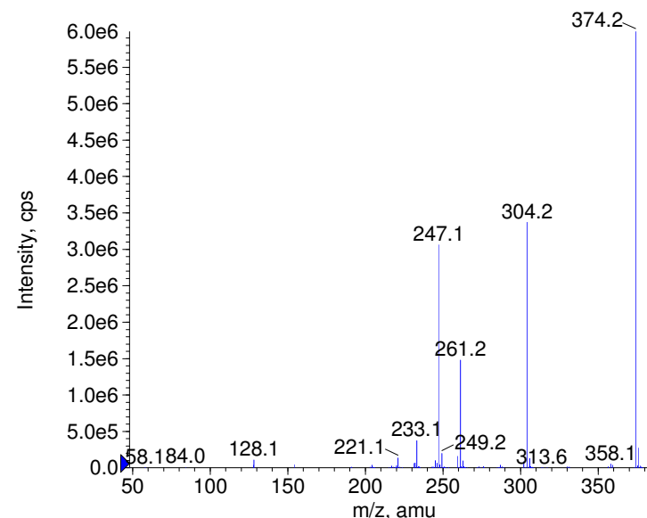
+ Bunazosin Prec(374.0) CE(99.0) RT(0.9)
