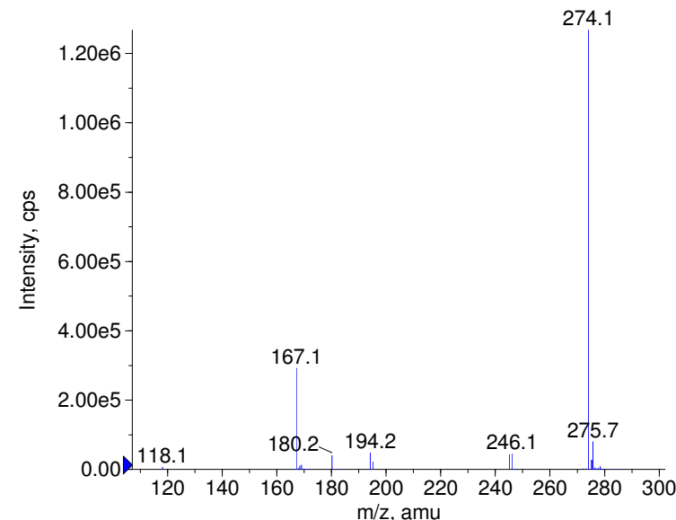
+ Brompheniramine Prec(319.0) CE(99.0) RT(0.8)
