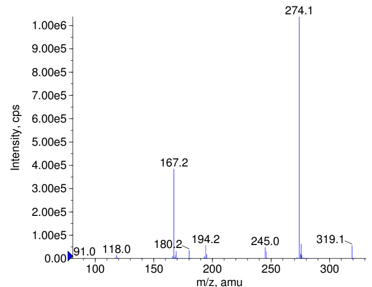
+ Brompheniramine Prec(319.0) CE(99.0) RT(0.8)
