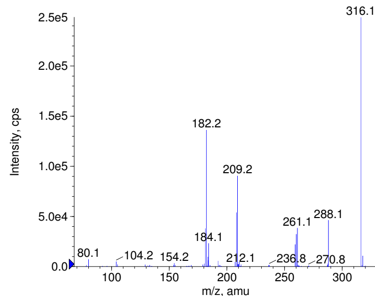
■ + Bromazepam Prec(316.0) CE(99.0) RT(0.8)
