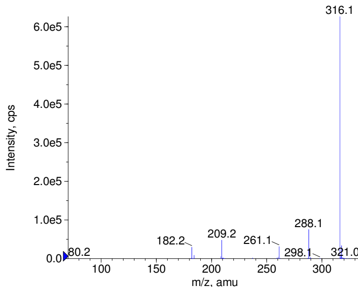
■ + Bromazepam Prec(316.0) CE(50.0) RT(0.8)
