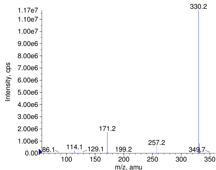
+ Bornaprine Prec(330.0) CE(50.0) RT(0.8)
