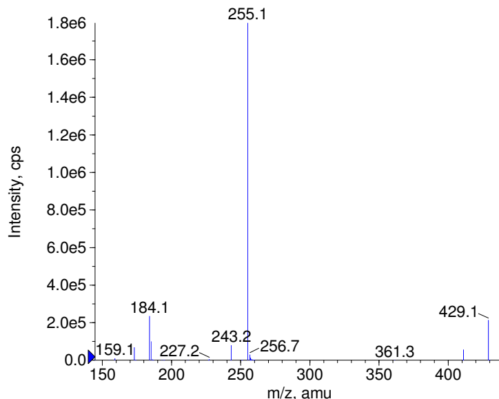
■ - Bicalutamide Prec(429.0) CE(-50.0) RT(1.2)
