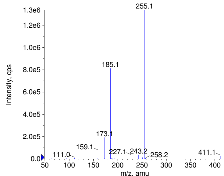
■ - Bicalutamide Prec(429.0) CE(-99.0) RT(1.2)
