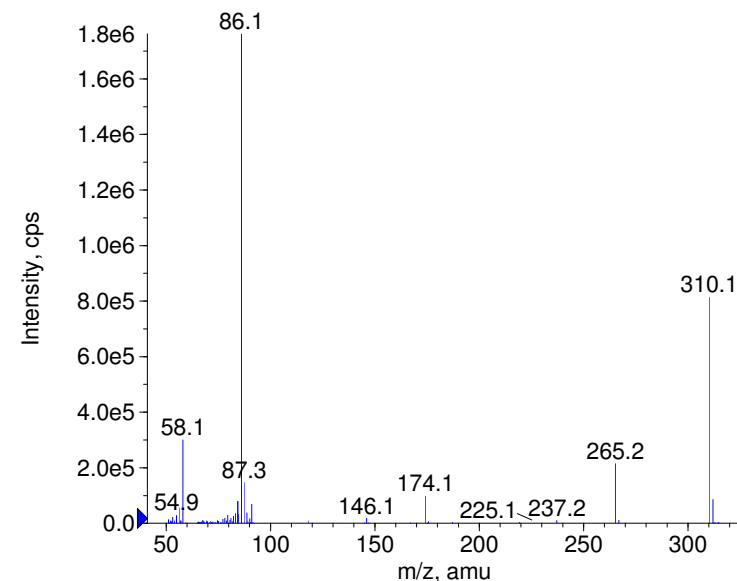
+ Benzydamine Prec(310.0) CE(99.0) RT(0.9)
