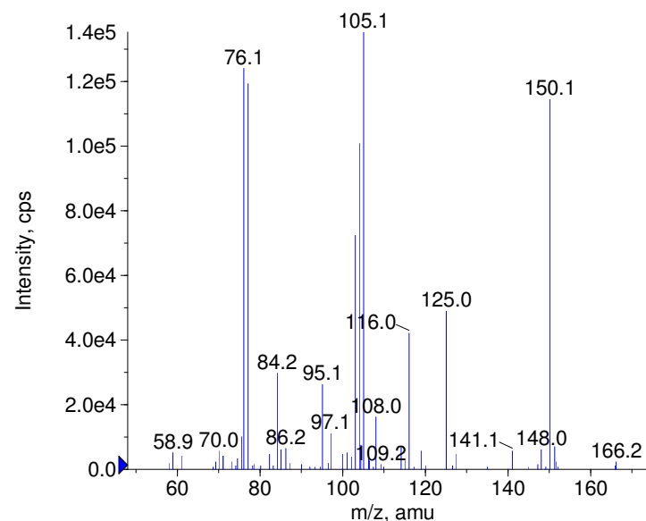
+ Bensultap Prec(432.0) CE(50.0) RT(0.9)
