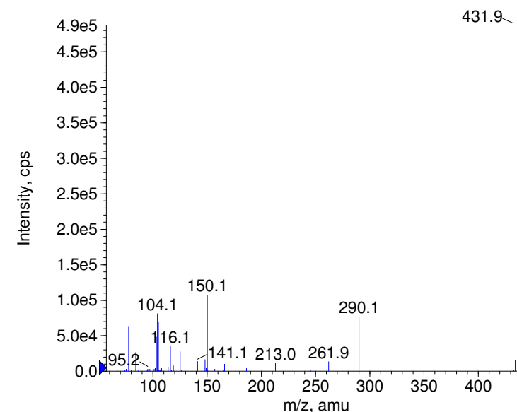
+ Bensultap Prec(432.0) CE(99.0) RT(0.9)
