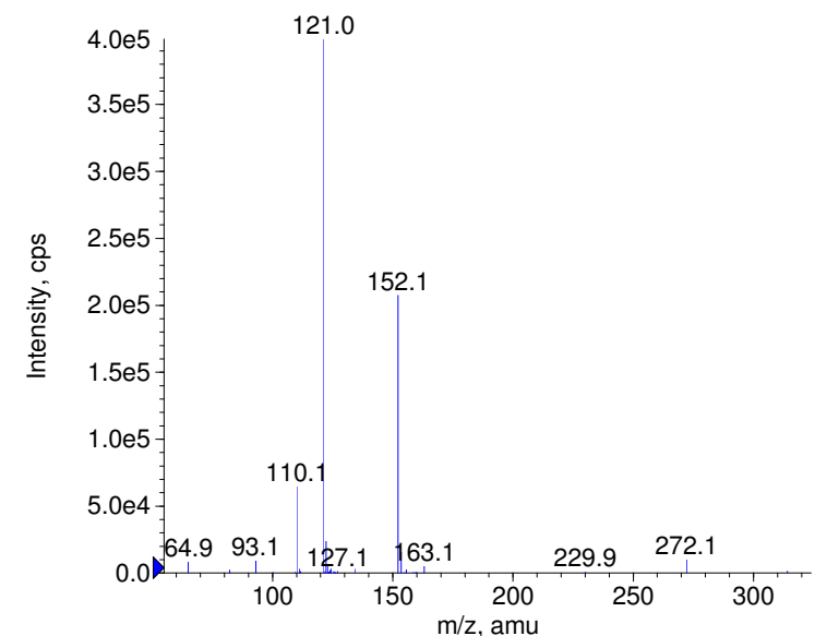
+ Benorilate Prec(314.0) CE(99.0) RT(1.0)
