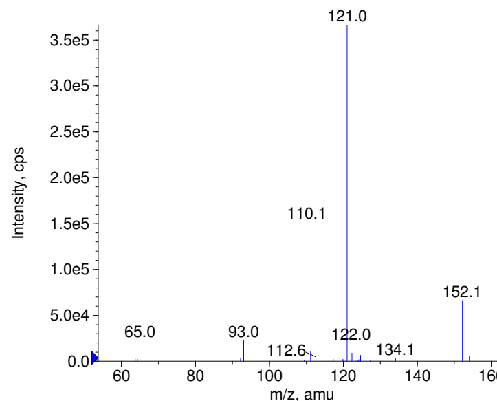
+ Benorilate Prec(314.0) CE(50.0) RT(1.0)
