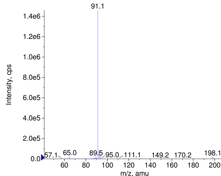
+ Beclamide Prec(198.0) CE(99.0) RT(1.2)
