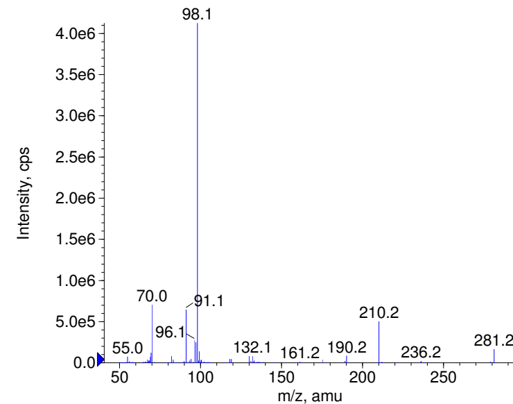
+ Bamipin Prec(281.0) CE(99.0) RT(0.9)
