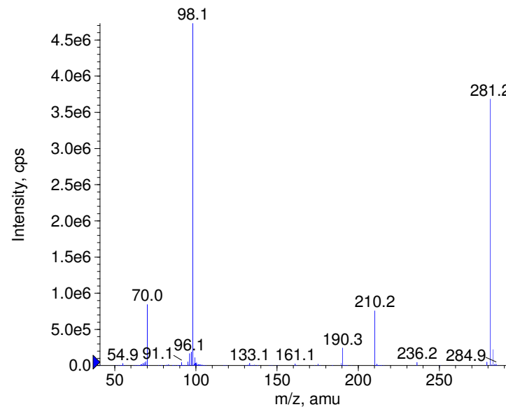
+ Bamipin Prec(281.0) CE(50.0) RT(0.9)
