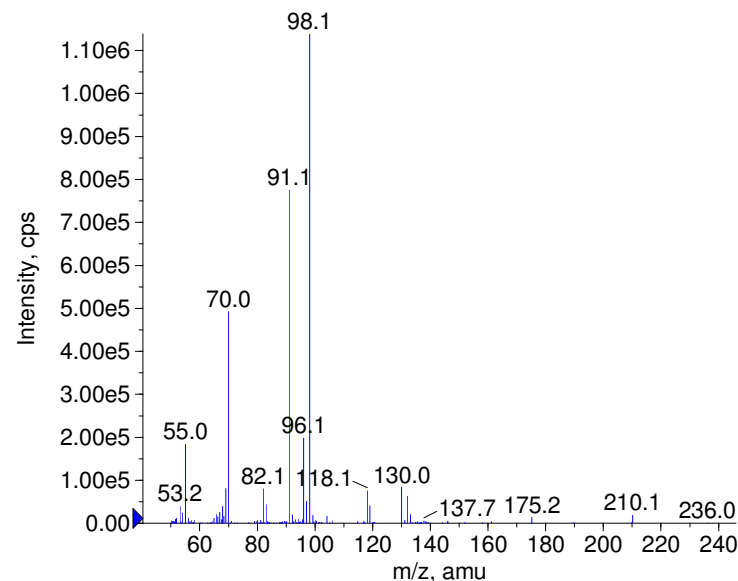
+ Bamipin Prec(281.0) CE(50.0) RT(0.9)
