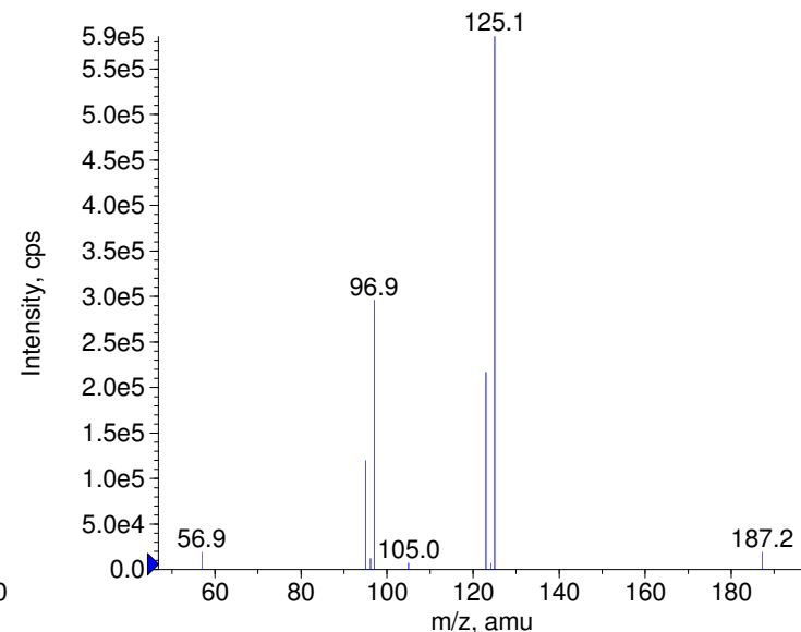
■ - Azelaic Acid Prec(187.0) CE(-99.0) RT(0.9)
