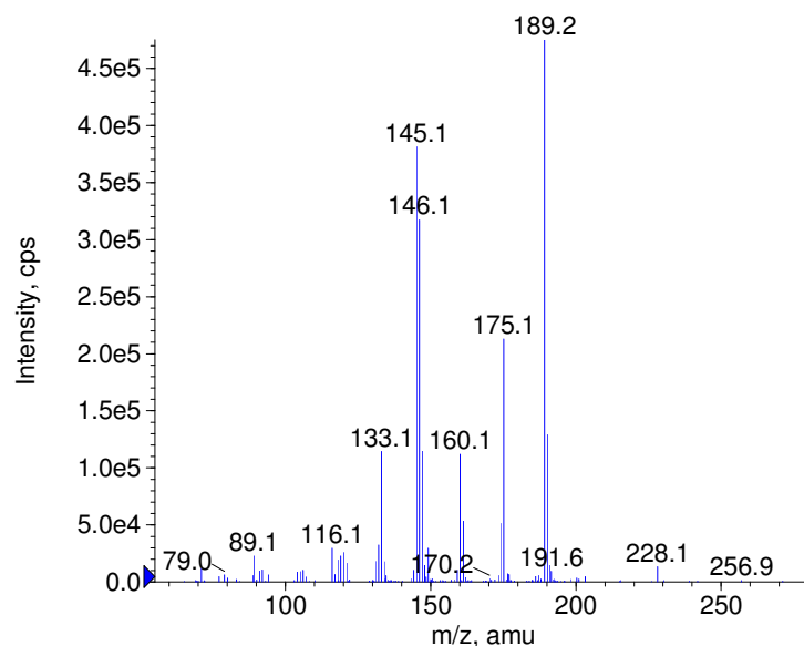
+ Azapropazone Prec(301.0) CE(50.0) RT(0.9)
