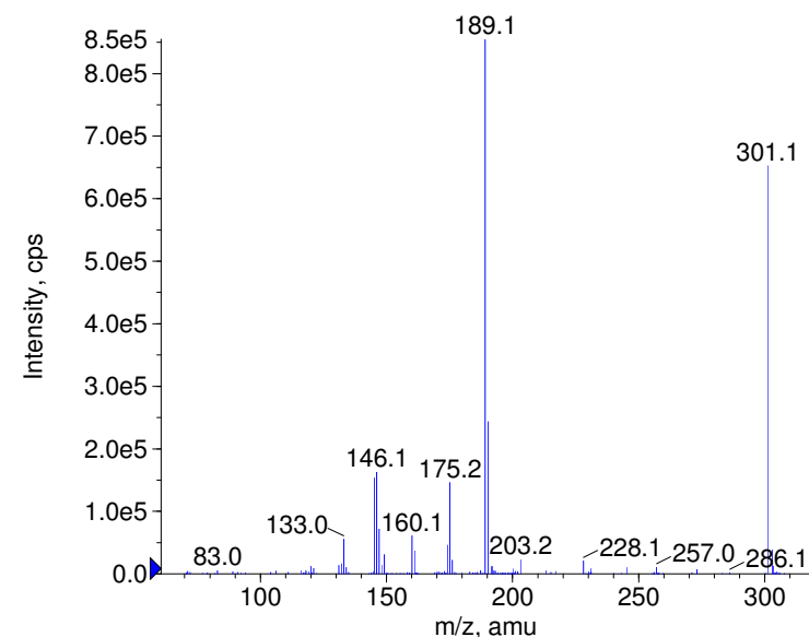
+ Azapropazone Prec(301.0) CE(99.0) RT(0.9)
