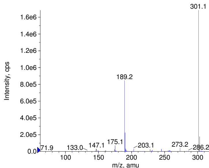
+ Azapropazone Prec(301.0) CE(50.0) RT(0.9)
