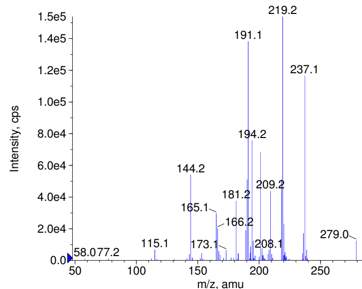
■ + Amprolium Prec(279.0) CE(99.0) RT(3.5)
