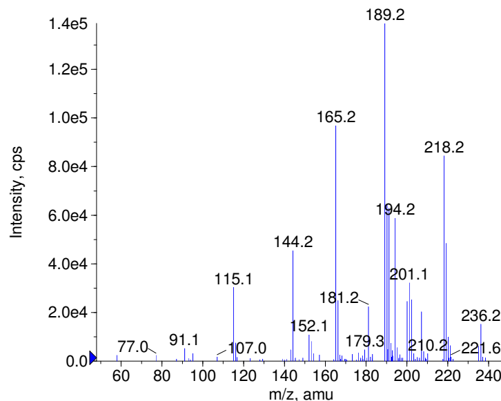
■ + Amprolium Prec(279.0) CE(50.0) RT(3.5)
