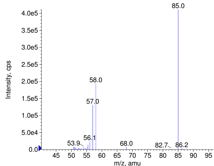
■ + Amitrole Prec(85.0) CE(99.0) RT(0.7)
