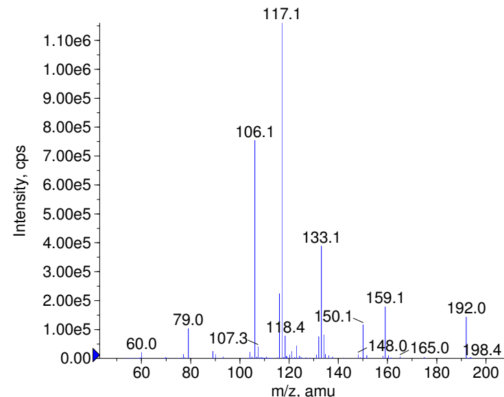
+ Amiphenazole Prec(192.0) CE(99.0) RT(0.8)
