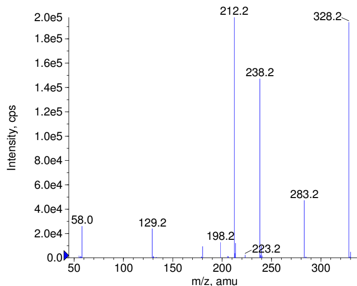
■ + Aminopromazine Prec(328.0) CE(50.0) RT(0.7)
