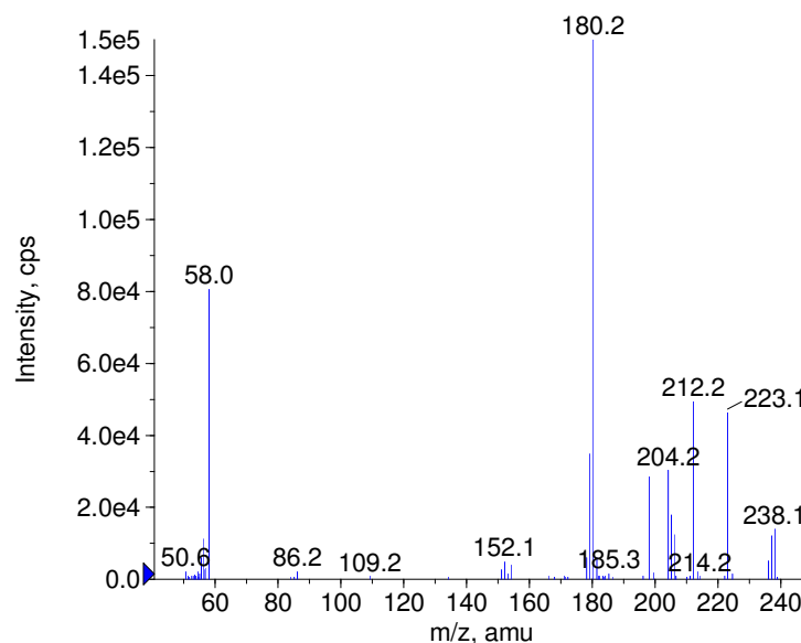
■ + Aminopromazine Prec(328.0) CE(50.0) RT(0.7)
