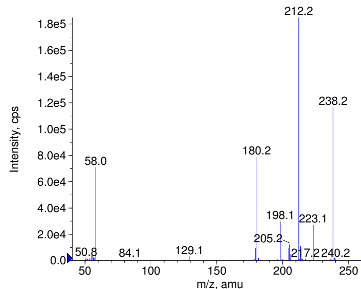
■ + Aminopromazine Prec(328.0) CE(99.0) RT(0.8)
