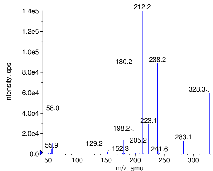
■ + Aminopromazine Prec(328.0) CE(99.0) RT(0.8)
