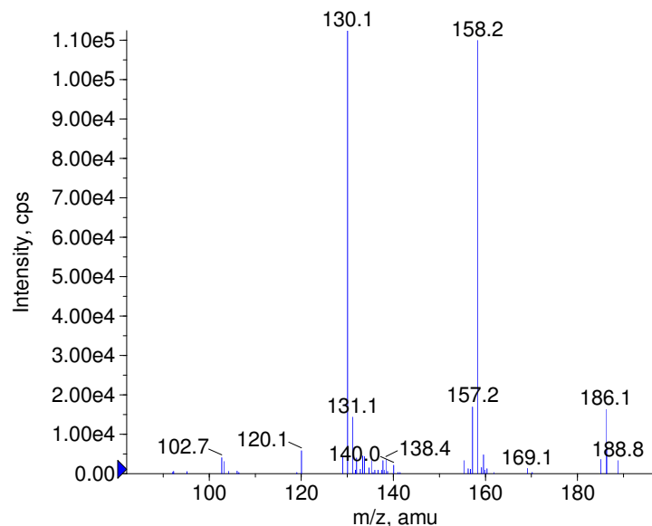
+ Aminodantrolene Prec(285.0) CE(50.0) RT(0.9)
