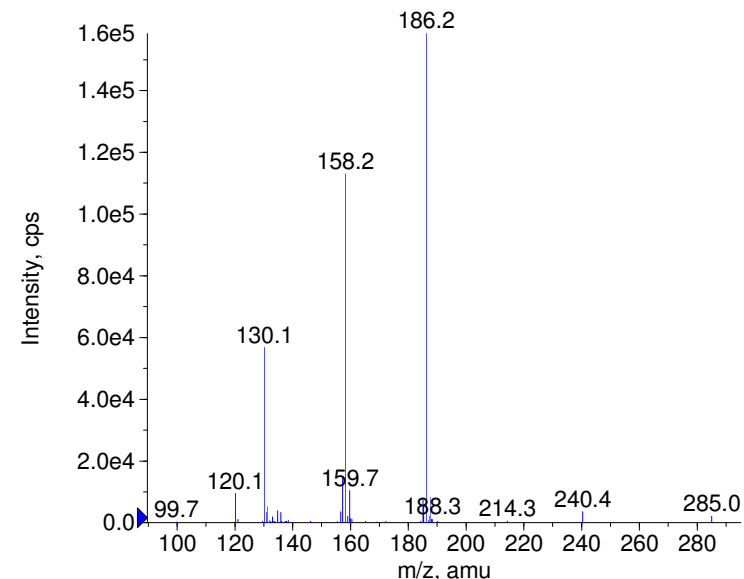
+ Aminodantrolene Prec(285.0) CE(99.0) RT(0.9)
