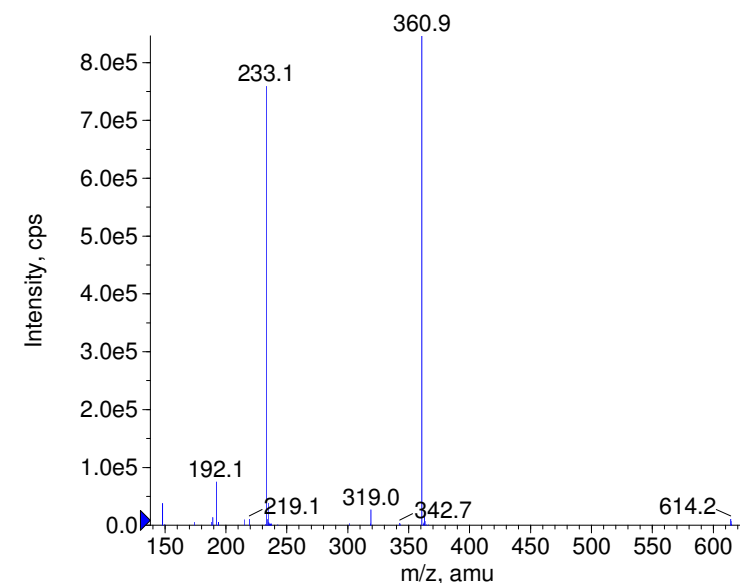
+ Amidotrizoic Acid Prec(615.0) CE(99.0) RT(1.0)
