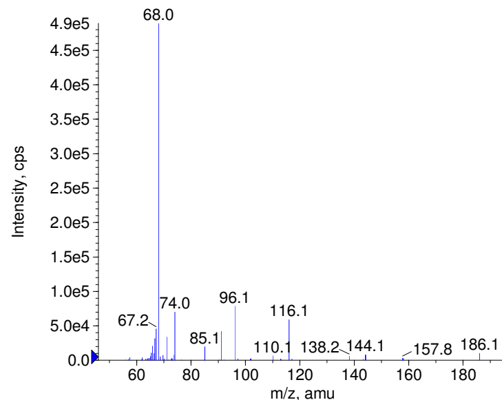
+ Ametryn Prec(228.0) CE(50.0) RT(1.2)
