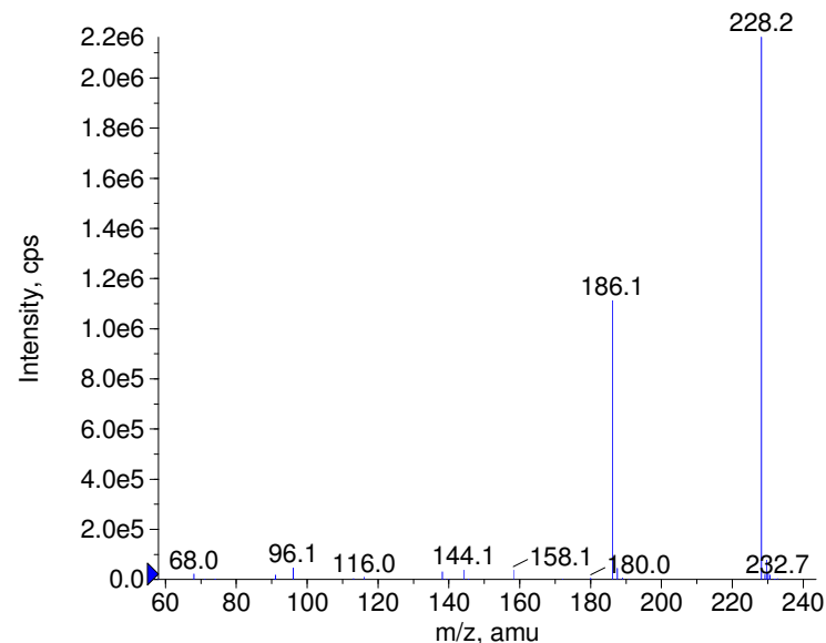
+ Ametryn Prec(228.0) CE(50.0) RT(1.2)
