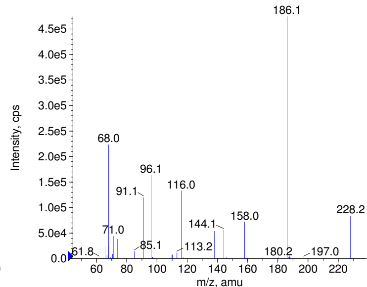
+ Ametryn Prec(228.0) CE(99.0) RT(1.2)
