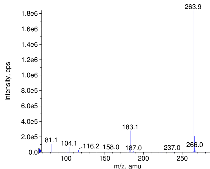
+ Ambroxol Prec(379.0) CE(50.0) RT(0.8)
