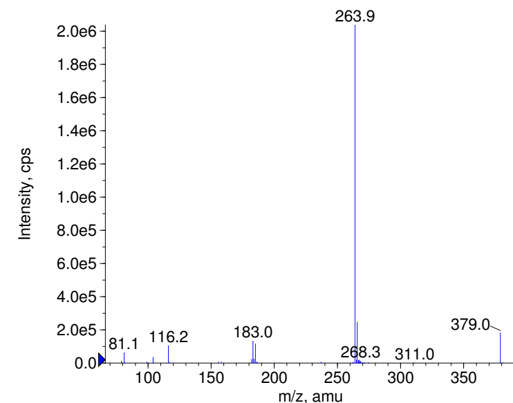
+ Ambroxol Prec(379.0) CE(99.0) RT(0.8)
