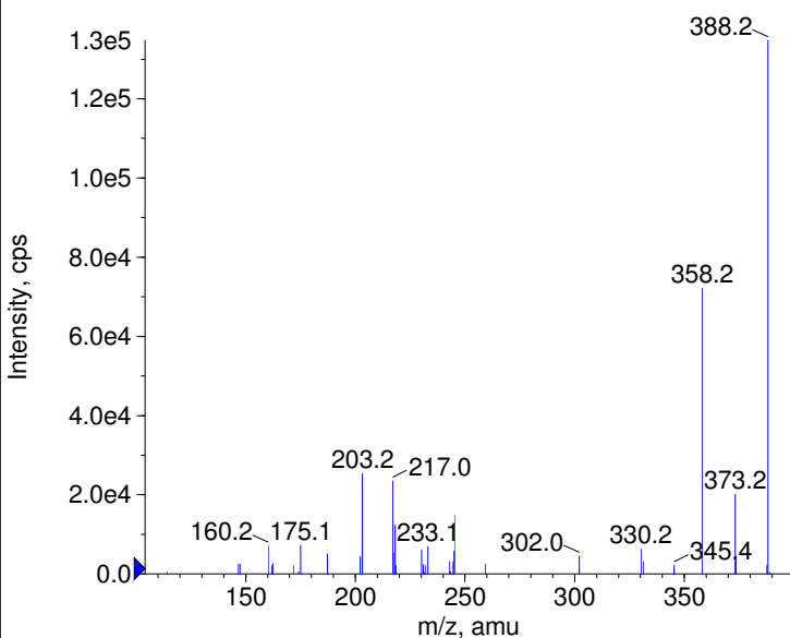
■ - Alfuzosine Prec(388.0) CE(-99.0) RT(1.0)
