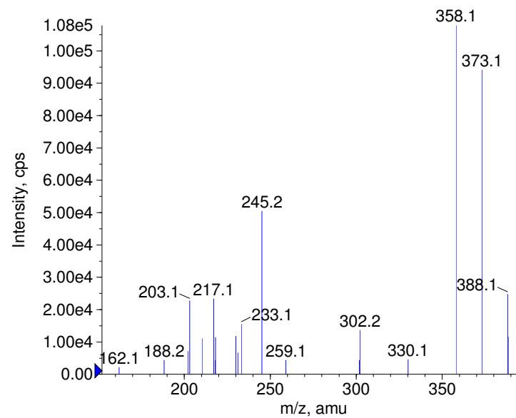
■ - Alfuzosine Prec(388.0) CE(-35.0) RT(0.9)
