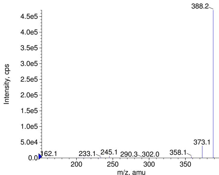
■ - Alfuzosine Prec(388.0) CE(-50.0) RT(0.9)
