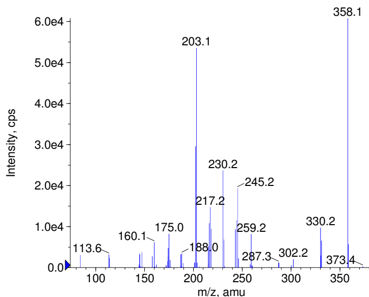
■ - Alfuzosine Prec(388.0) CE(-50.0) RT(0.9)
