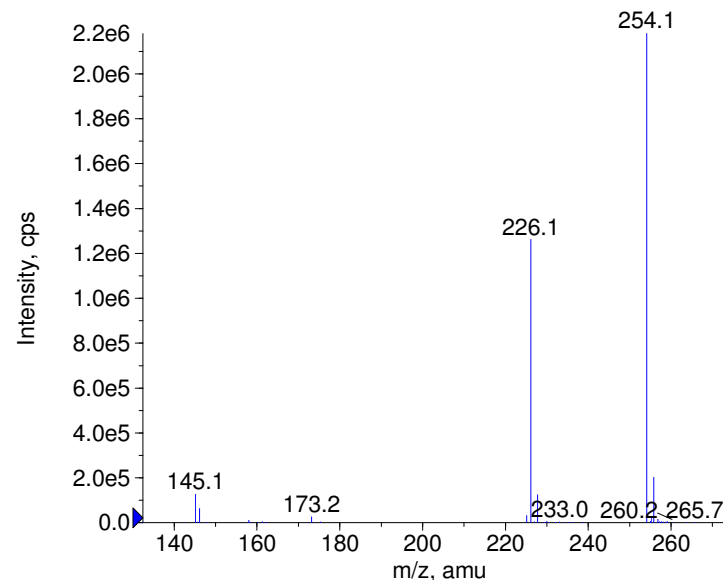
+ Actinoquinol Prec(254.0) CE(50.0) RT(0.9)
