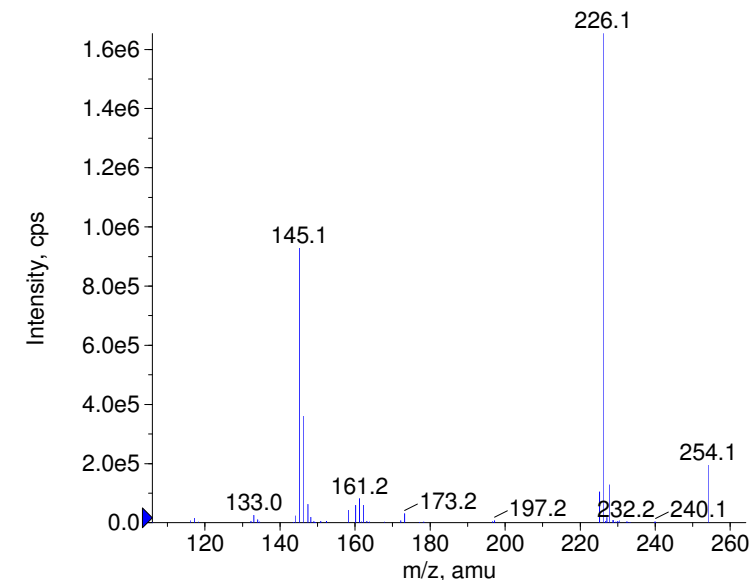
+ Actinoquinol Prec(254.0) CE(99.0) RT(0.9)
