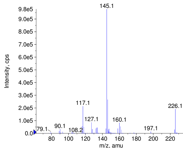
+ Actinoquinol Prec(254.0) CE(50.0) RT(0.9)
